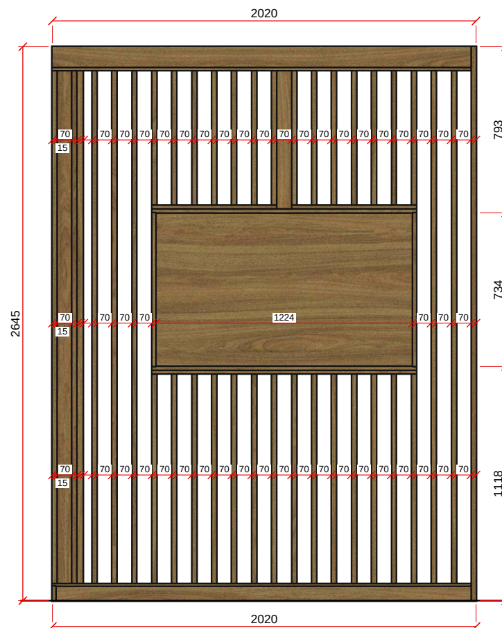
DIVISORIA - ESC. 1:25
